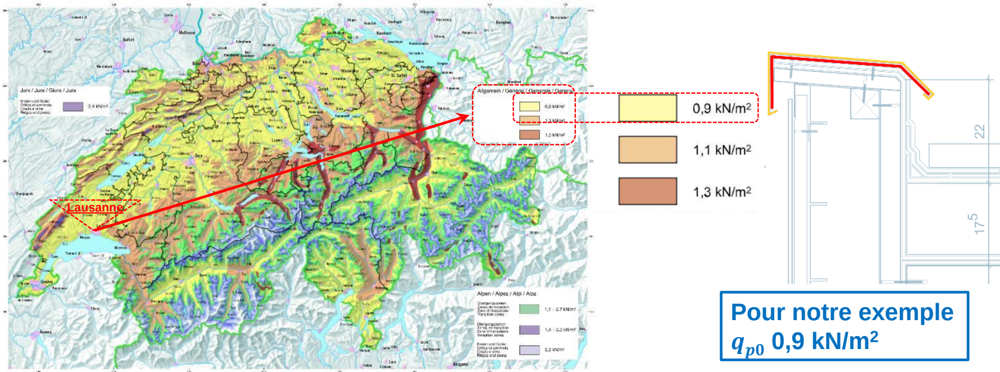
Annexe E (normative) Valeur de référence de la pression dynamique
