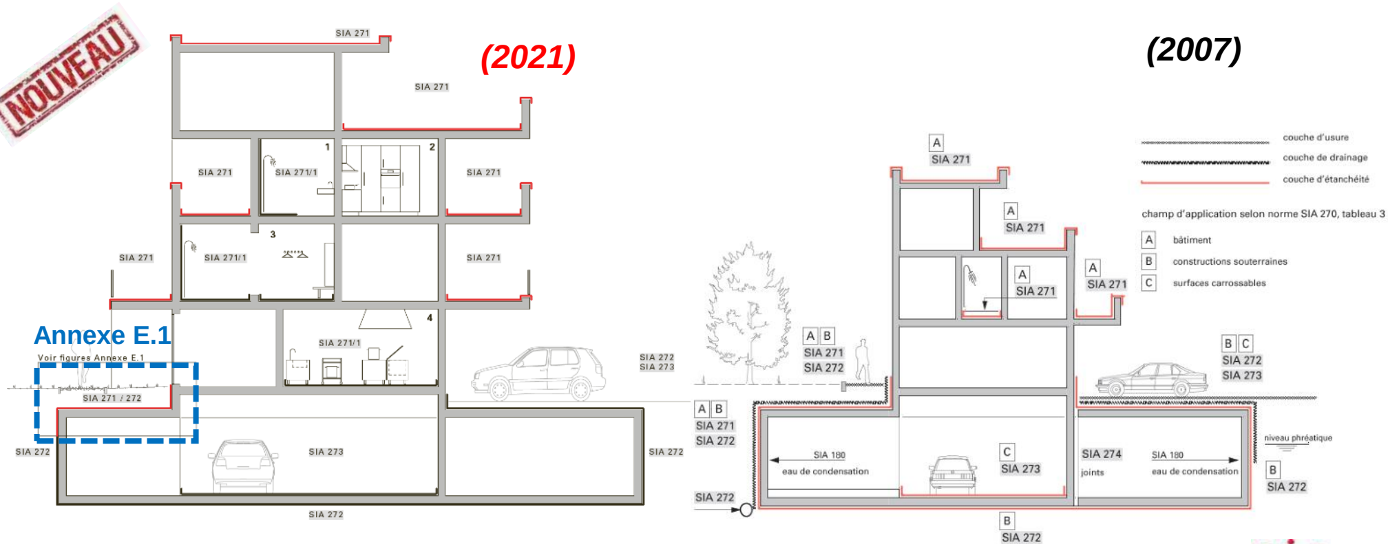
Figure 1 Croquis général
